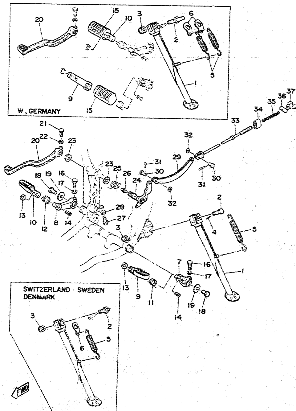
Fig. 21 STAND · FOOTREST · BRAKE PEDAL
