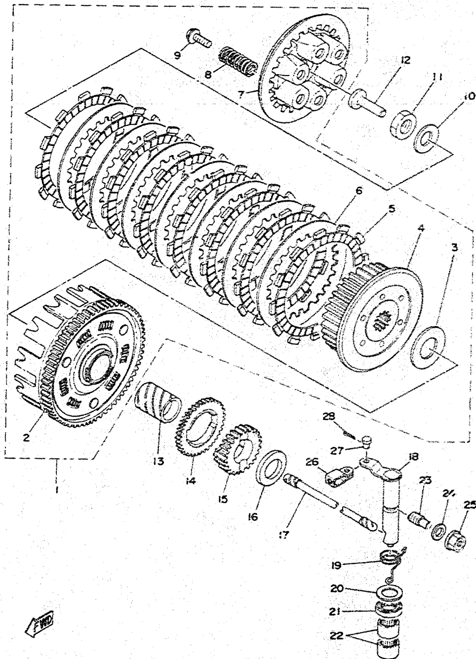
Fig. 10 CLUTCH
