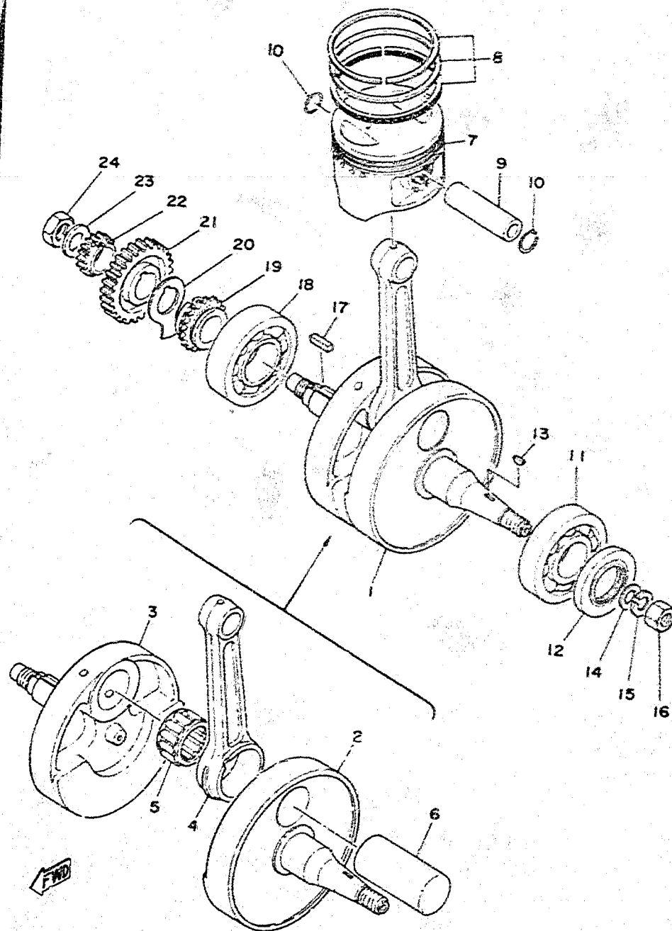
Fig. 3 CRANK · PISTON
