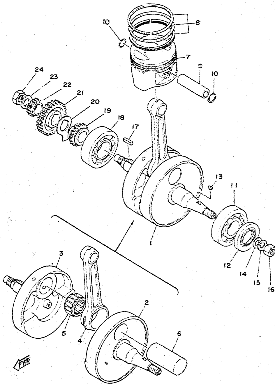
Fig. 3 CRANK · PISTON
