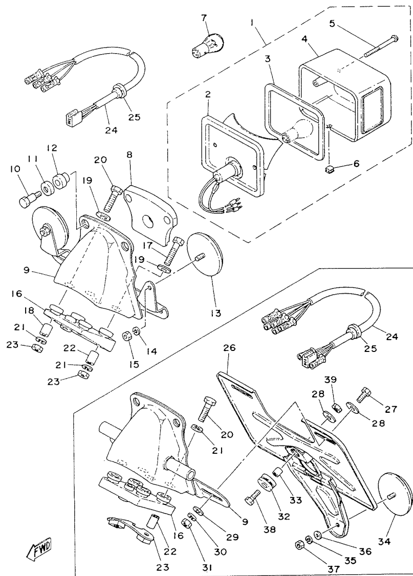
Fig. 35 FEU ARRIERE
