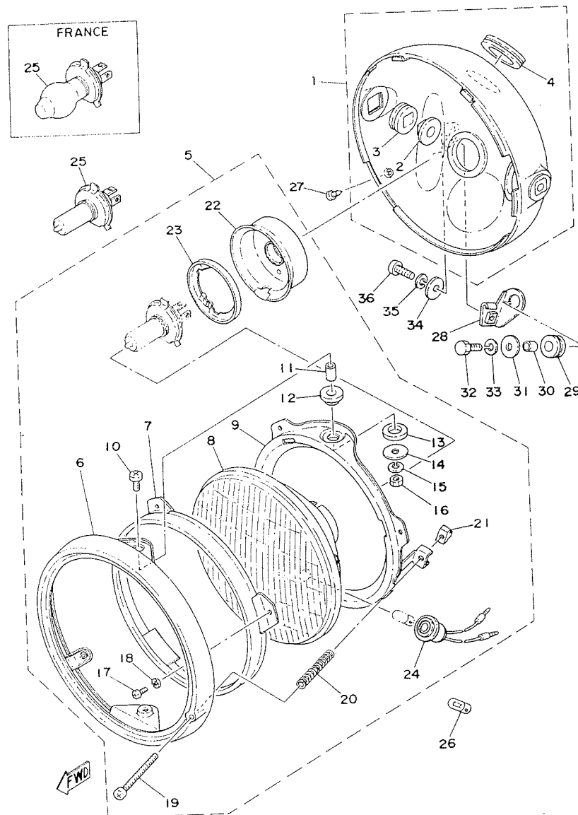
Fig. 32 PHARE 1
