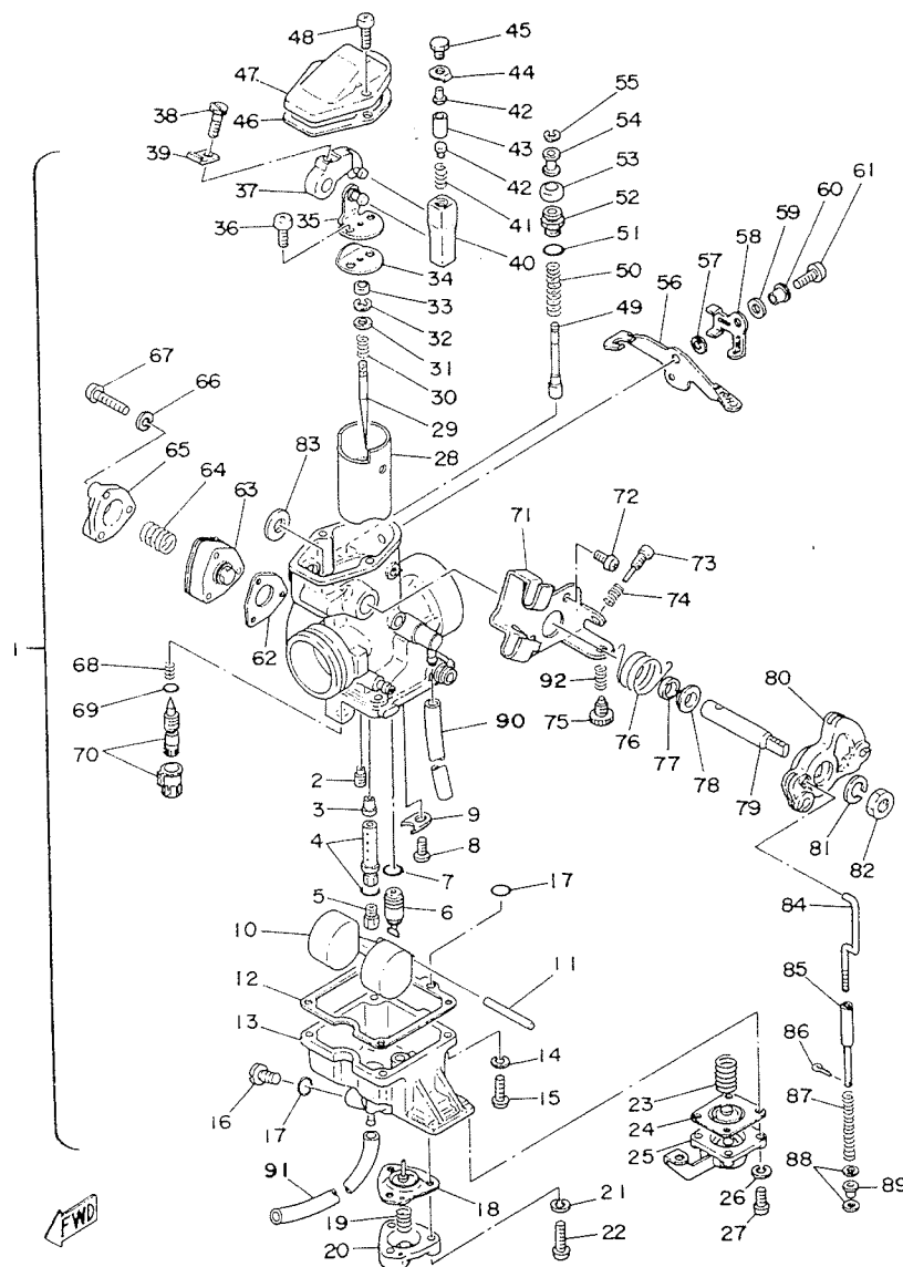
Fig. 15 CARBURATEUR
