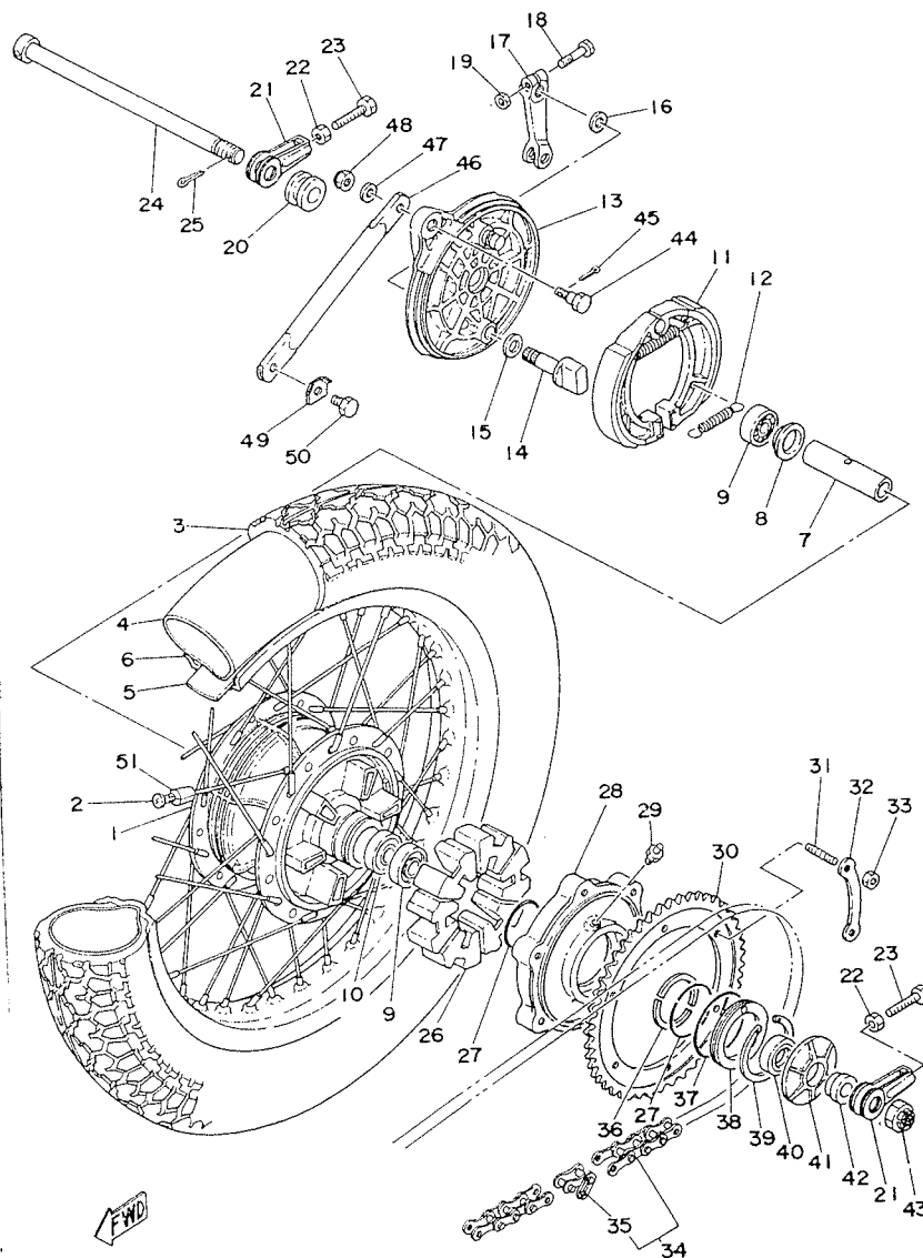
Fig. 31 ROUE ARRIERE
