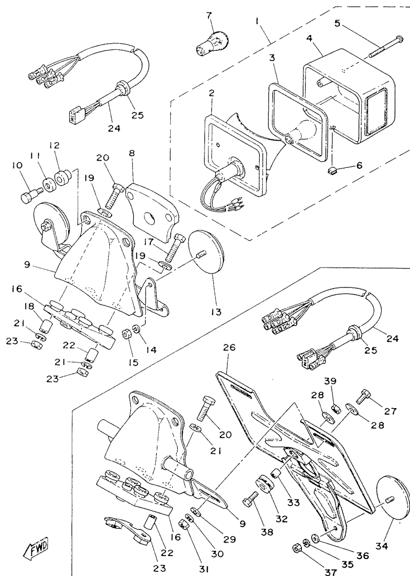
Fig. 35 FEU ARRIERE
