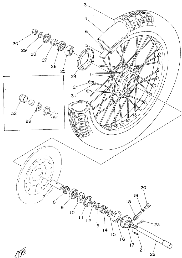
Fig. 29 ROUE AVANT
