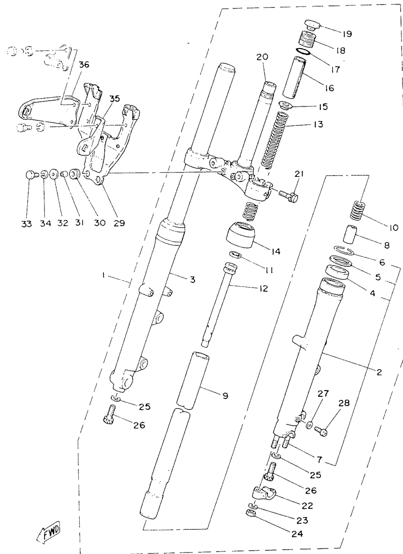
Fig. 23 FOURCHE AVANT
