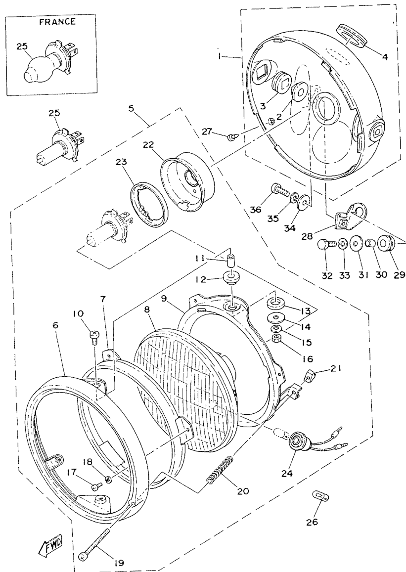
Fig. 32 PHARE 1
