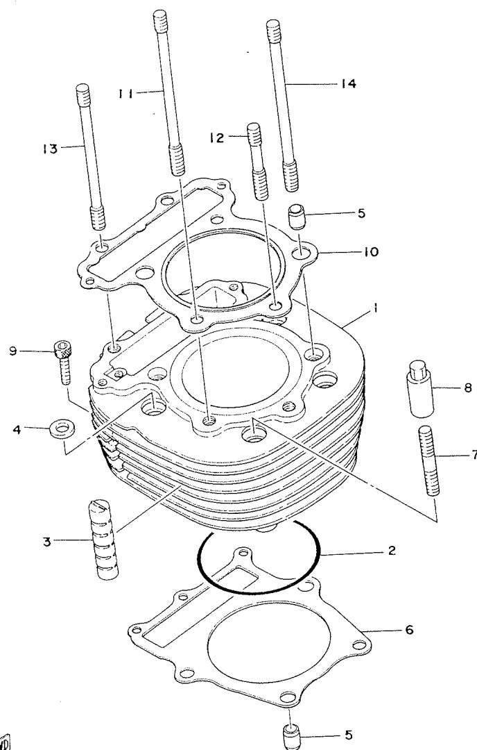
Fig. 2 CYLINDRE
