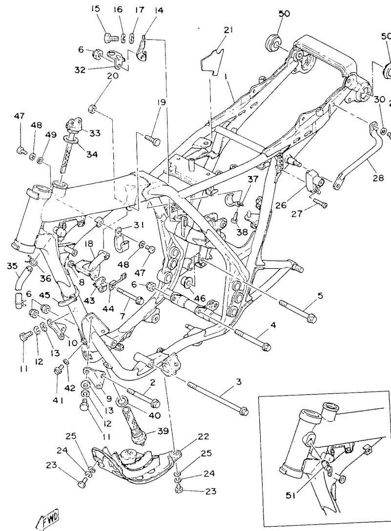
Fig. 18 CADRE
