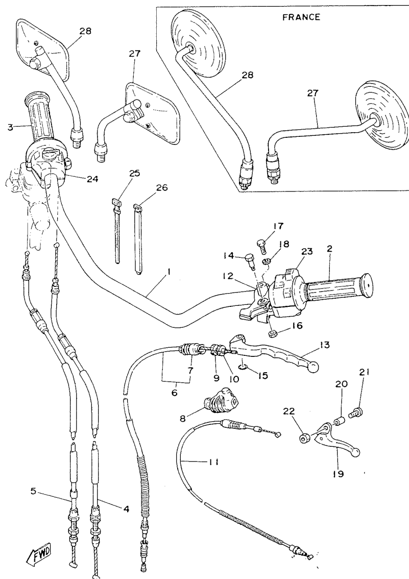
Fig. 25 GUIDON • CABLES
