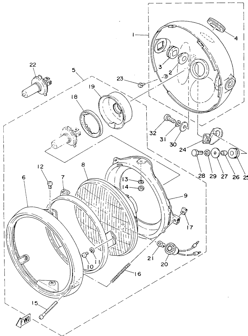
Fig. 33 PHARE 2 (L'ANGLETERRE)
