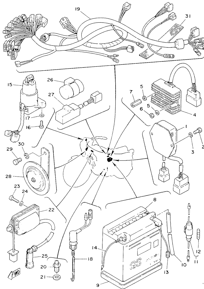
Fig. 37 PARTIE ELECTRIQUE
