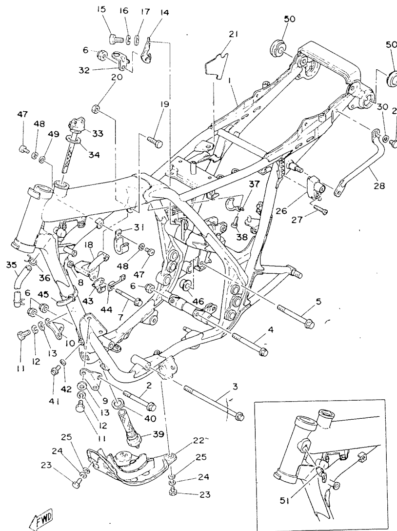
Fig. 18 CADRE
