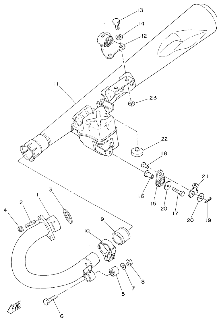
Fig. 16 ECHAPPEMENT
