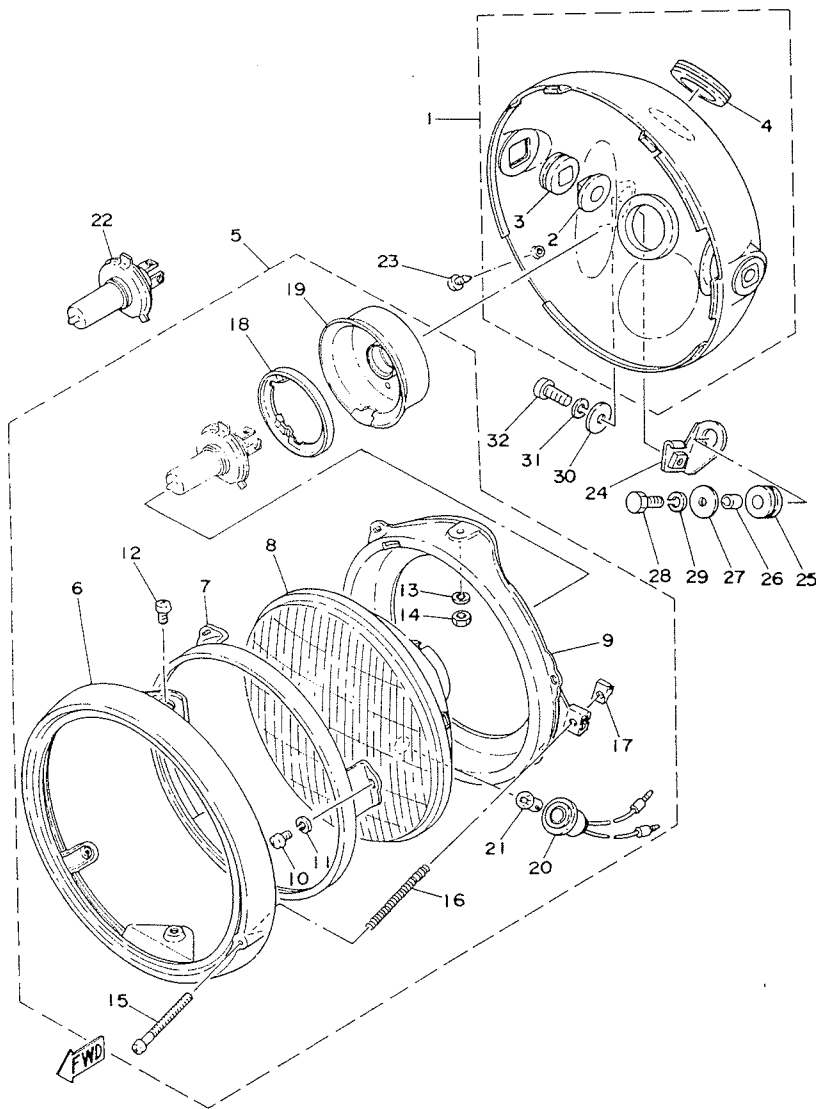
Fig. 33 PHARE 2 (L'ANGLETERRE)
