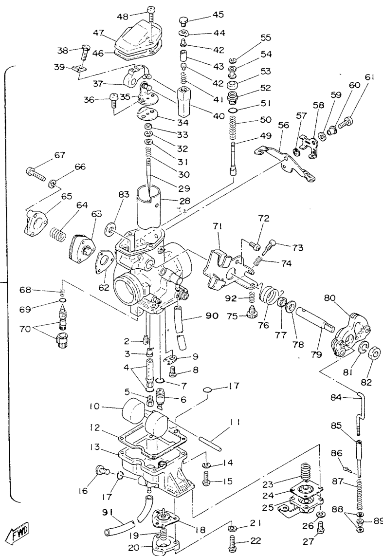
Fig. 15 CARBURATEUR
