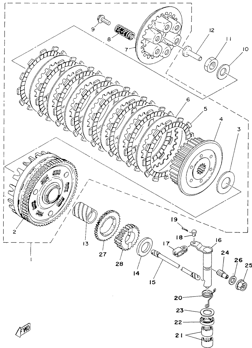
Fig. 9 EMBRAYAGE
