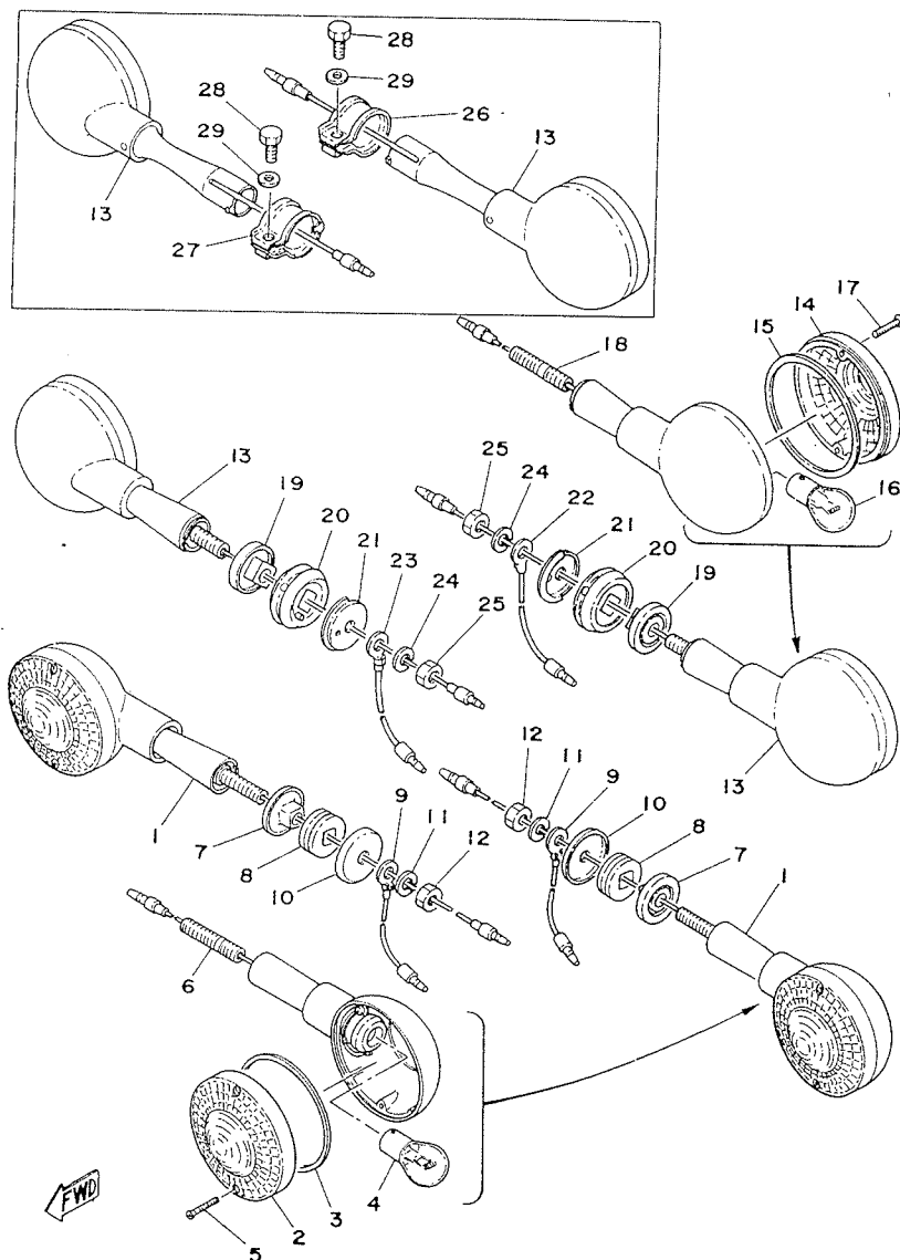
Fig. 36 CLIGNOTEUR
