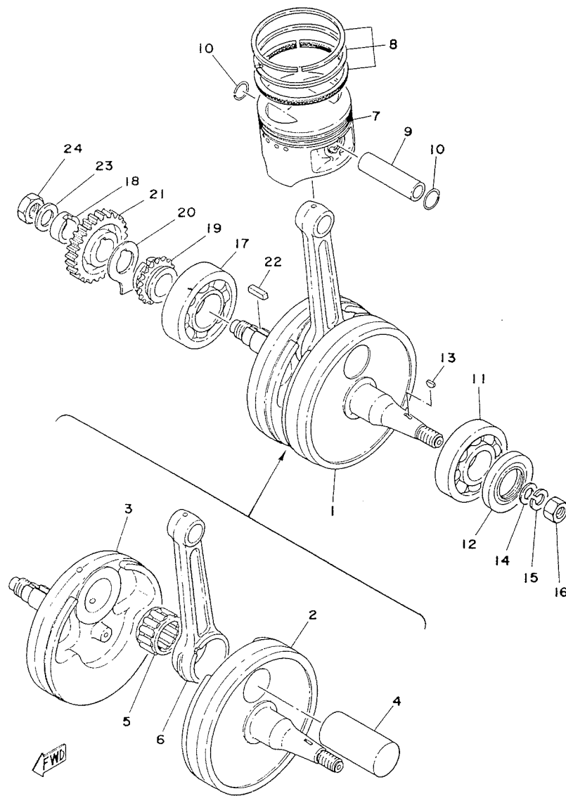
Fig. 3 VILEBREQUIN • PISTON
